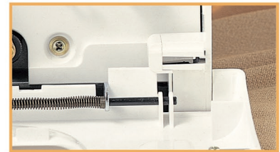
Veiligheidsschakelaar Voor Geopend Frontdeksel
